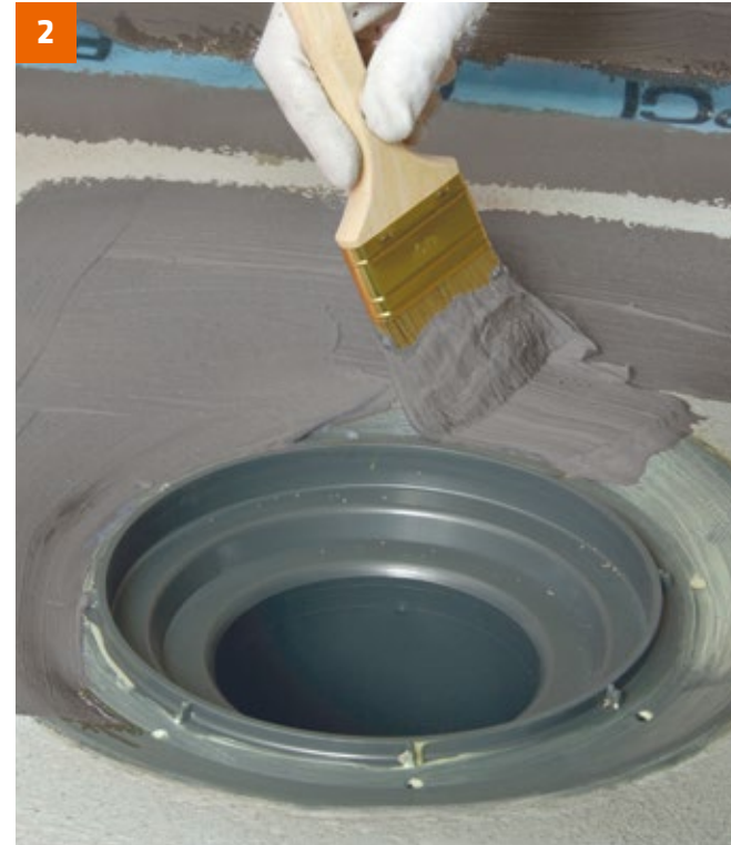
PCI Seccoral 1K / 2K Rapid vorlegen ...
