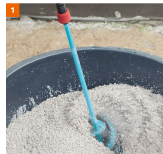
Drainmörtel PCI Epoxigrund 390 und PCI Quarzsand DM 1 bis 4 anrühren.
