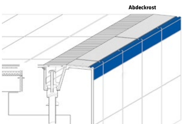
System Finland II: Schräger, strandähnlicher Beckenrand mit Handfasse, abgedeckte Rinne mit Rinnenschale und Flüsterablauf SILENT 100. Besonders geeignet für Sport- und Wettkampfbecken.
