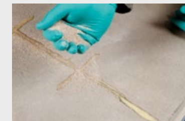
Angemischtes Gießharz in die Risse/Fugen oberflächenbündig eingießen, glatt abziehen und mit trockenem Quarzsand abstreuen.
