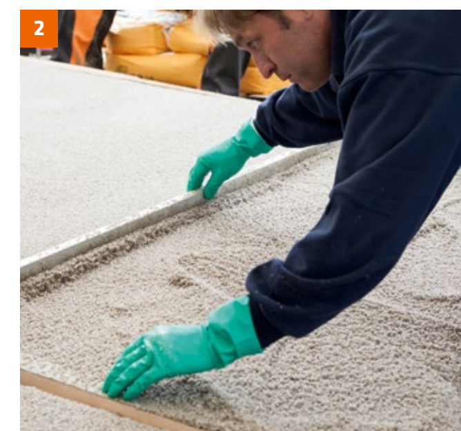
Die angerührte Mörtelmischung auftragen und über Lehren abziehen.
