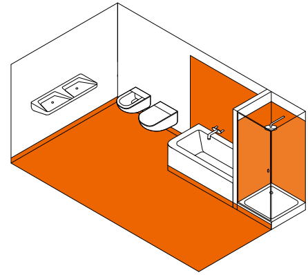
Häusliches Bad mit Badewanne ohne Brause und mit Duschtasse mit Duschabtrennung
