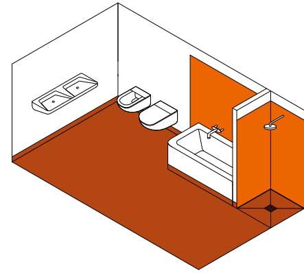
Häusliches Bad mit Badewanne ohne Brause und mit bodengleicher Dusche ohne Duschabtrennung
