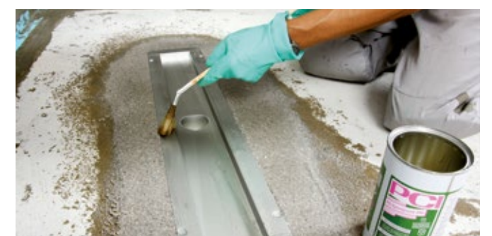
Nach dem Einbetten der Ablaufrinne im hoch wasserbeanspruchten Bereich mit Epoxidharz-Mörtel wird der Klebeflansch mit der Epoxidharz-Grundierung PCI Epoxigrund 390 oder PCI Elastoprimer Uni grundiert und im frischen Zustand mit feuergetrocknetem Quarzsand abgestreut.
