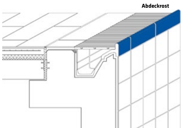
System Berlin: Hochliegende Überflutungskante als Handfasse, abgedeckte Rinne mit „weichem“ Einlauf. Für öffentliche Bäder und Sanierungen.
