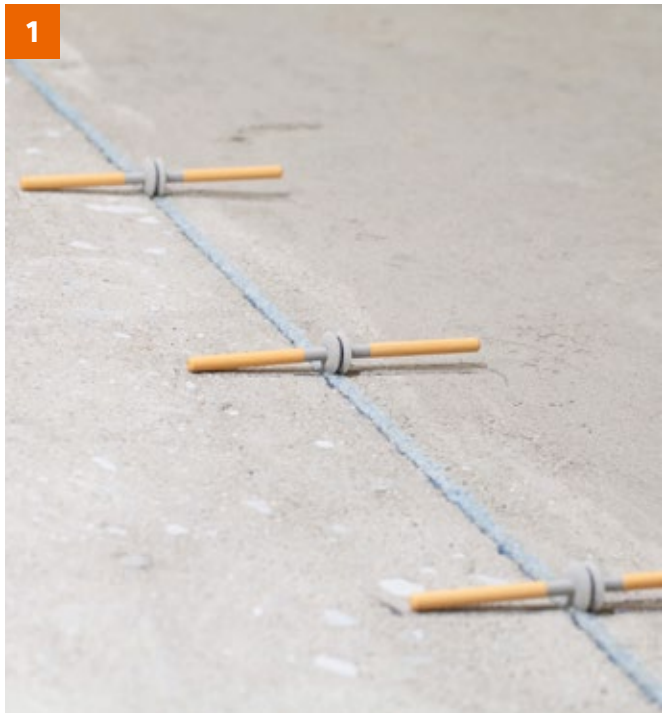
Die Dübel werden im Abstand von 20 bis 30 cm positioniert.
