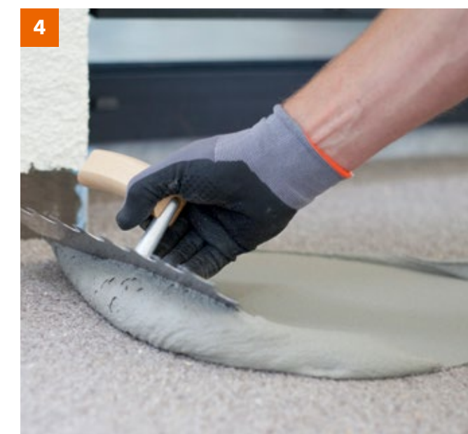
PCI Nanorapid vorlegen und als Kratzspachtelung ausführen.
