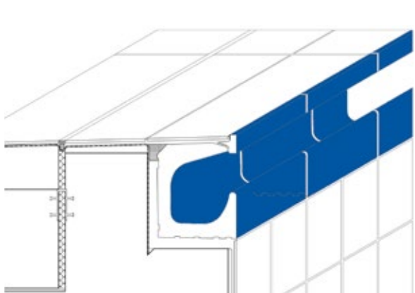
System Bamberg: Großer Rinnenstein mit Handfasse, Ablauf (Ø 75 mm), ohne Abdeckrost. Bei vielen Bäderarten einsetzbar.
