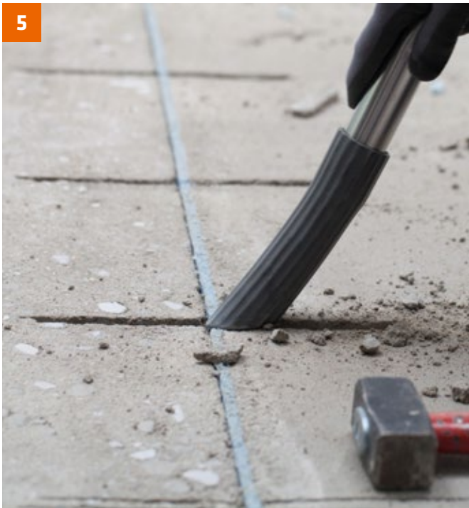
... und lose Estrichreste mittels Industriestaubsauger abgesaugt.
