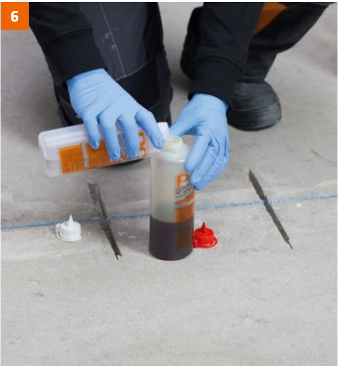
Sind die Nuten so weit vorbereitet, werden die beiden Komponenten von PCI Apogel SH zusammengeschüttet ...
